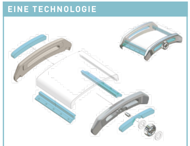
Kleben der Uhrgläser auf einem Rahmen von Christophe Claret
